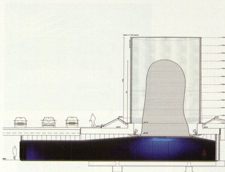
PLANTA Y SECCIÓN
